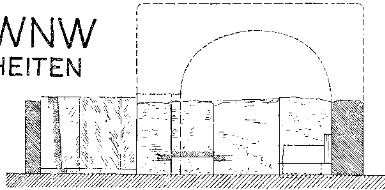
LANGS-SCHNITT DURCH DEN ZIEGEL-VORBAU P-Q
