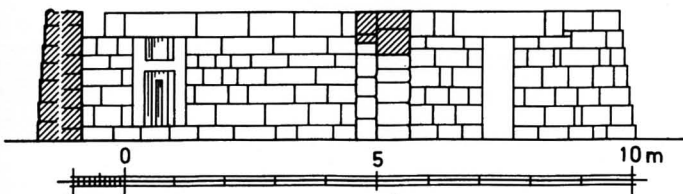
D 38, Ostansicht
