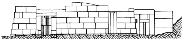
D 203, Ostansicht
