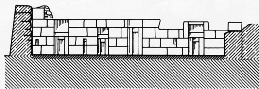
D 61, Schnitt SN
